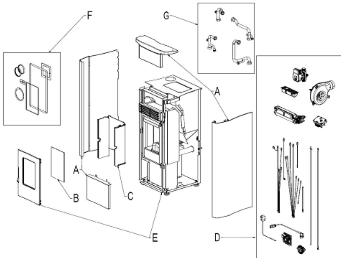
Fig. 1 - Geëxplodeerde tekening
